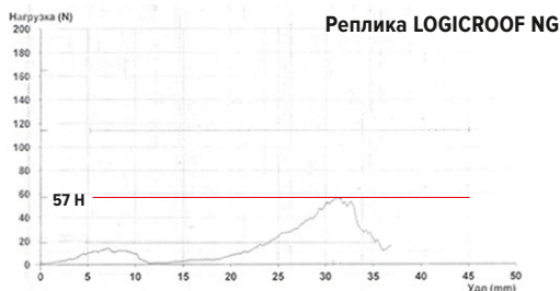
Прочность сварного шва на разрыв, Н/50мм
